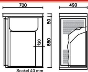
Maschinenteil EMA490 mit eingebauter Maschine und Becken
