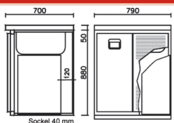
Maschinenteil EMA790R mit eingebauter Maschine und Becken
